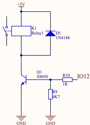
CH1继电器控制电路
