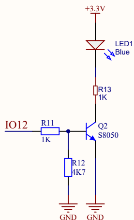
开关状态指示灯
