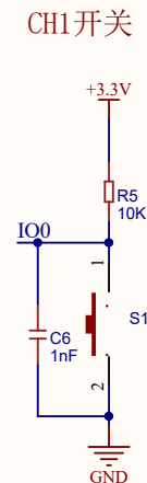
开关按键电路
