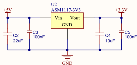
+3.3V电源电路
