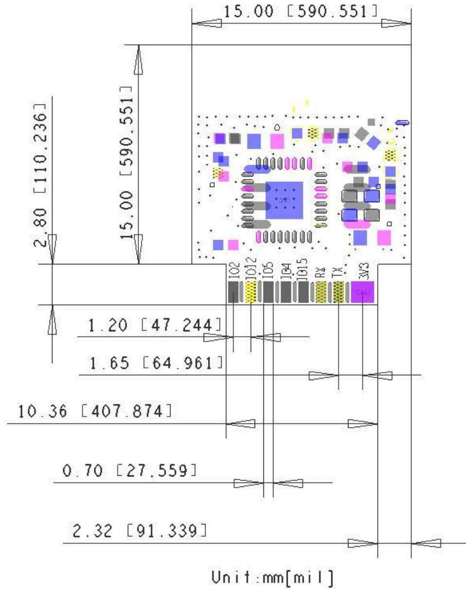
图 6 尺寸标注图
