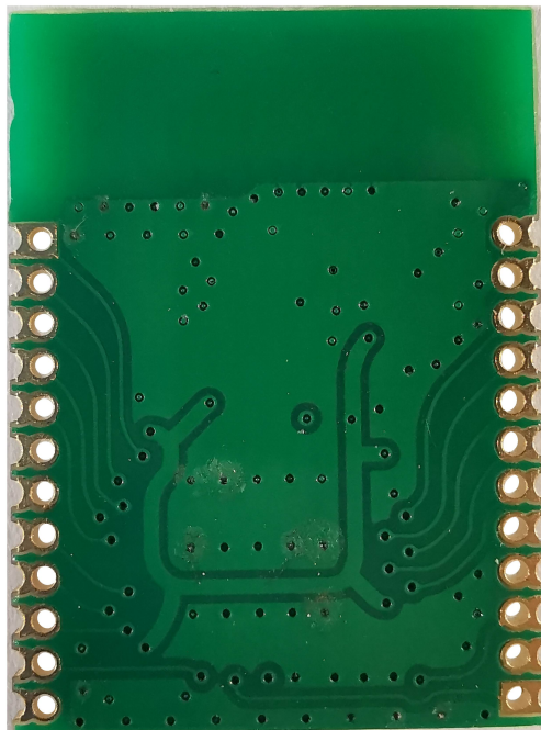
ZM-TH01 模块正面脚位图
